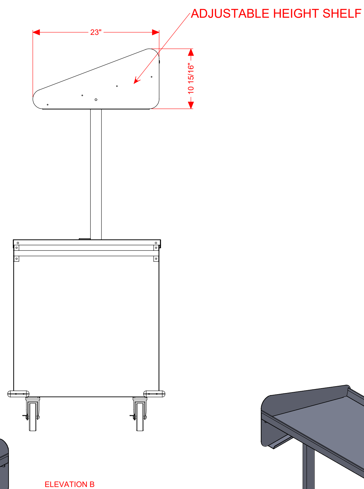
ELEVATION B
