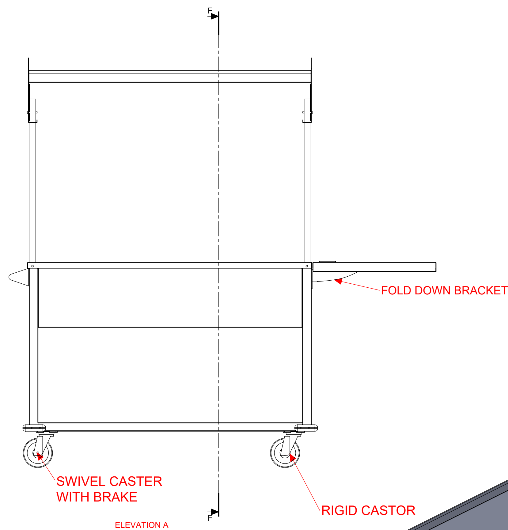
ELEVATION A
