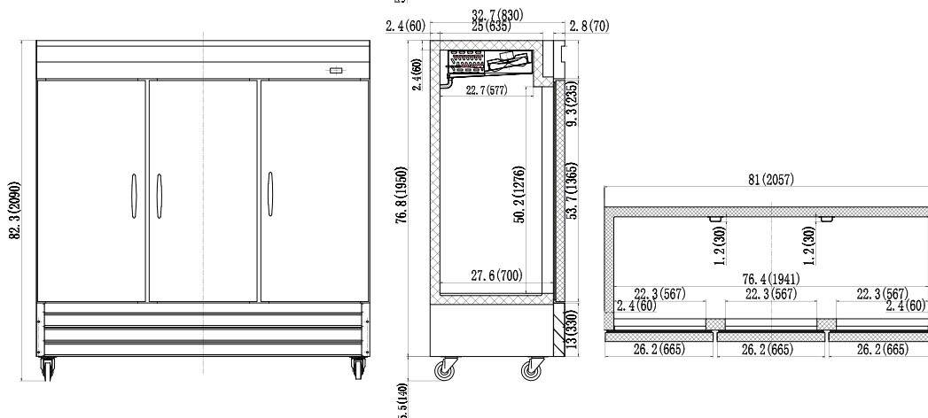
IB81F-DV
