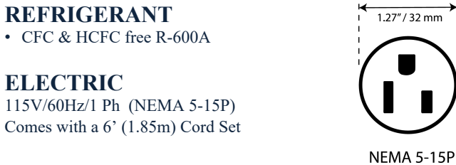
NEMA 5-15P
