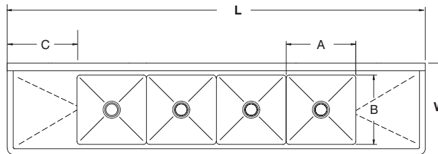
4 COMP - 2 DRBD
