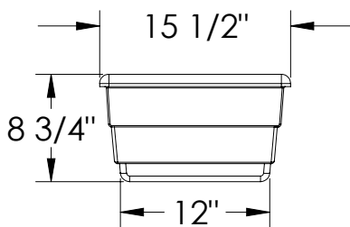
Lug Dimensions
