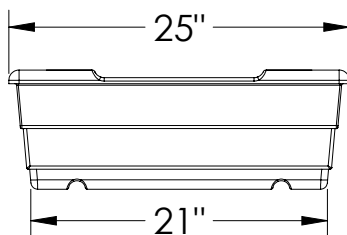
Lug Dimensions
